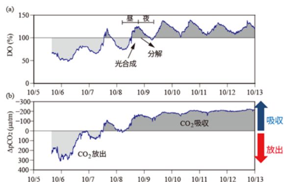
図 新西宮ヨットハーバーでのDOと \Delta p\text{CO}_2 の変動(2011年)
